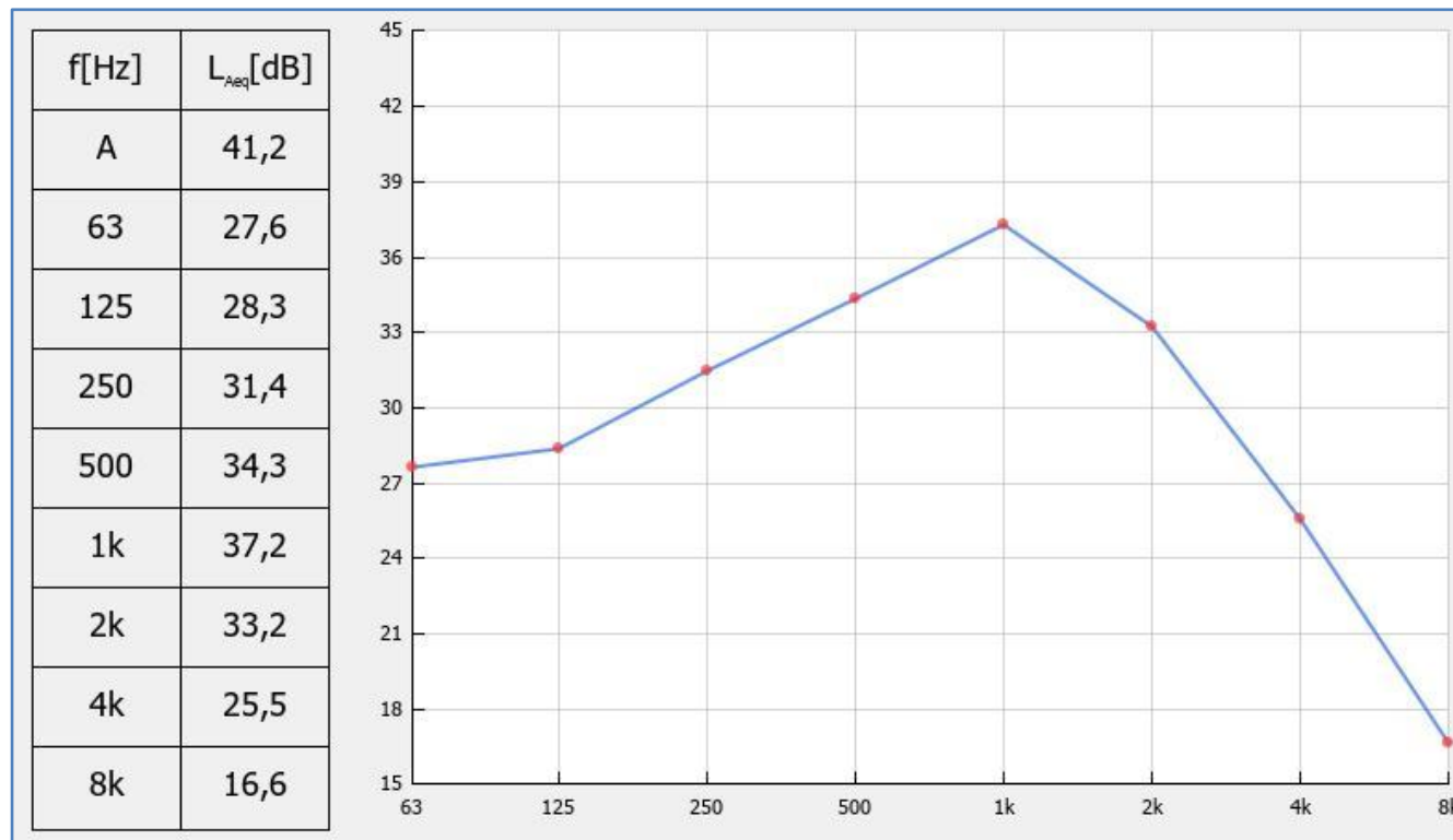
MM1 - Noćno merenje 2 - rezultati merenja
