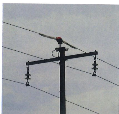
Прилог 1. Пример постављања пластичних покривки на изолаторе
