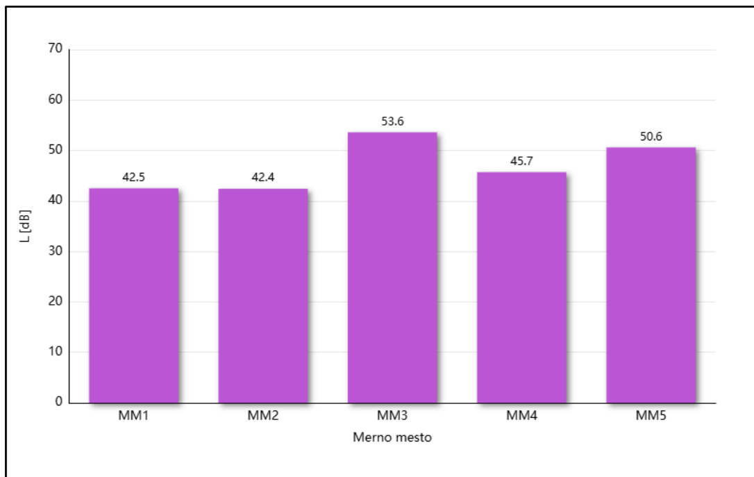
Grafik 5.10. - Noćni period merenja 2 - Ekvivalentni nivoi buke - decembar 2025. godine
