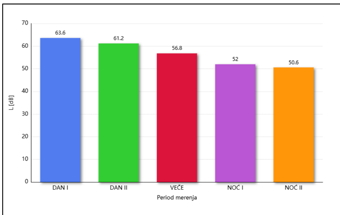
Grafik 5.5. - MM 5 ekvivalentni nivo buke za sve periode merenja - decembar 2025. godine
