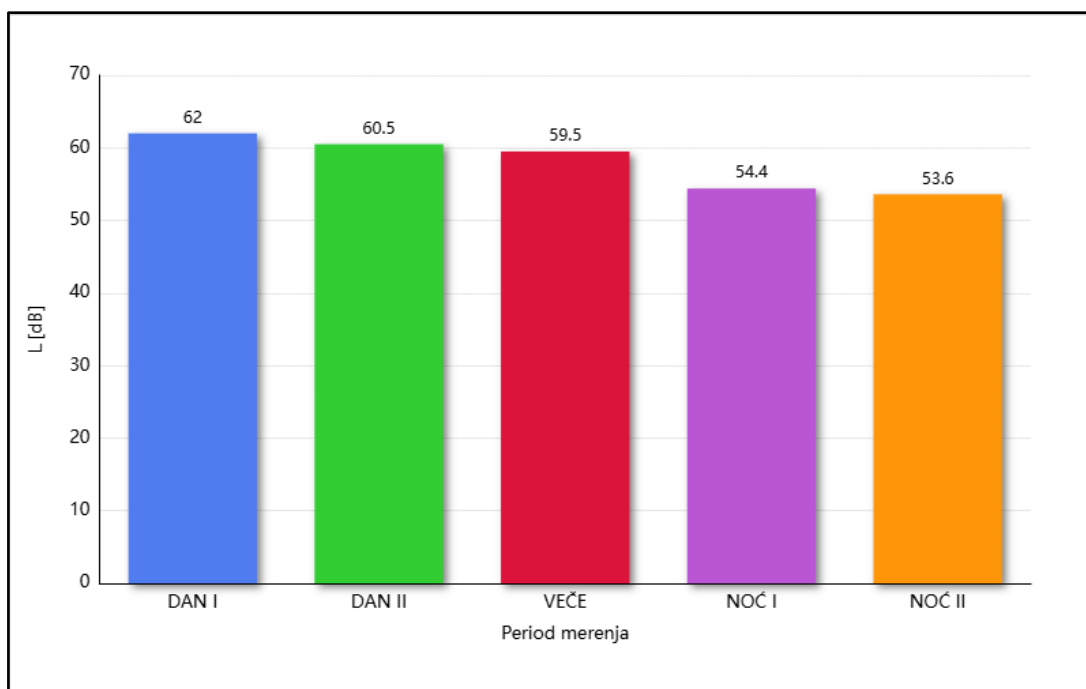
Grafik 5.3. - MM 3 ekvivalentni nivo buke za sve periode merenja - decembar 2025. godine
