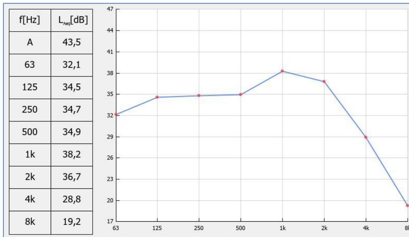
MM1 - Noćno merenje 1 - rezultati merenja
