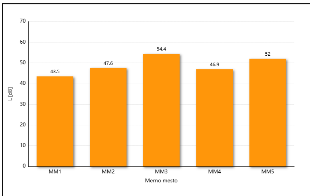
Grafik 5.9. - Noćni period merenja 1 - Ekvivalentni nivoi buke - decembar 2025. godine
