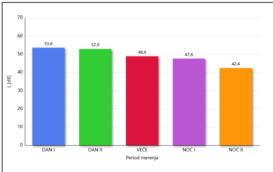
Grafik 5.2. - MM 2 ekvivalentni nivo buke za sve periode merenja - decembar 2025. godine
