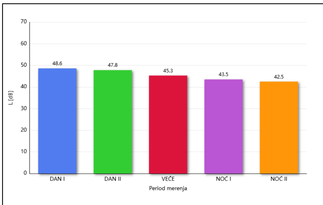
Grafik 5.1. - MM 1 ekvivalentni nivo buke za sve periode merenja - decembar 2025. godine
