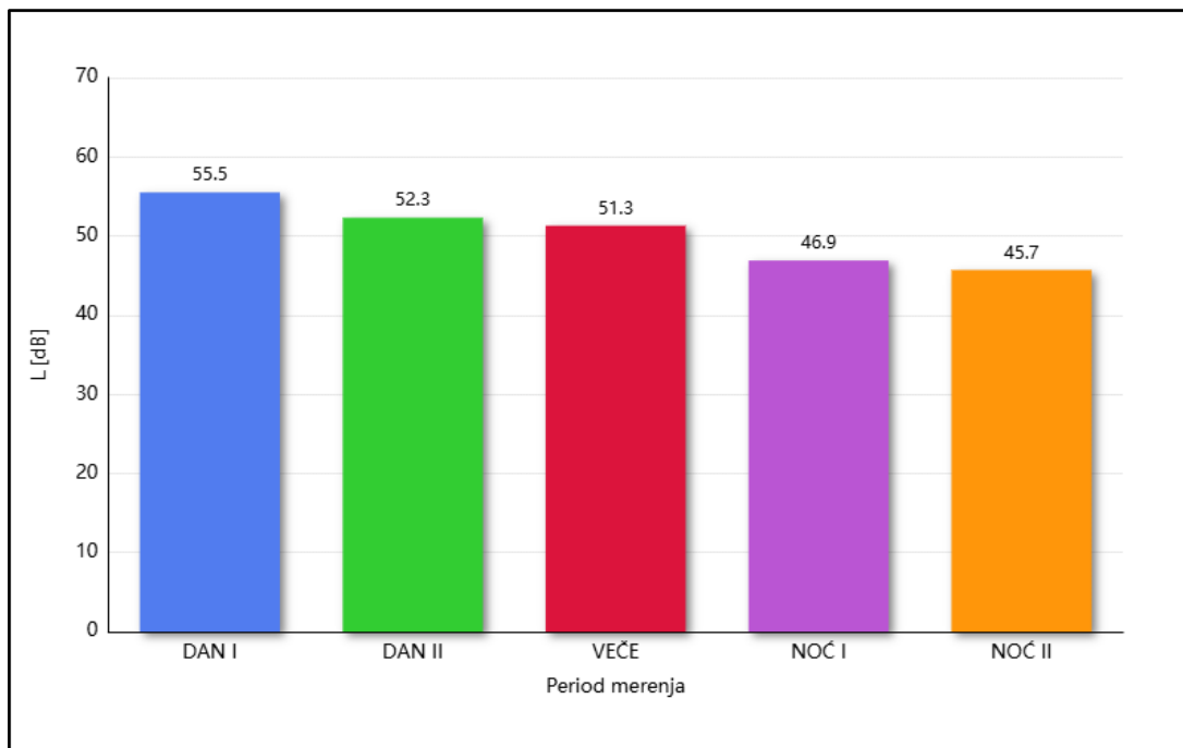
Grafik 5.4. - MM 4 ekvivalentni nivo buke za sve periode merenja - decembar 2025. godine
