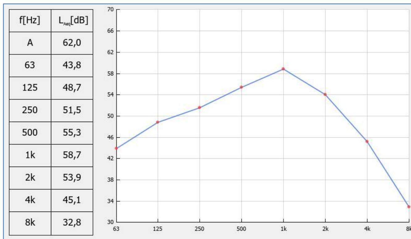
MM3 - Dnevno merenje 1 - rezultati merenja
