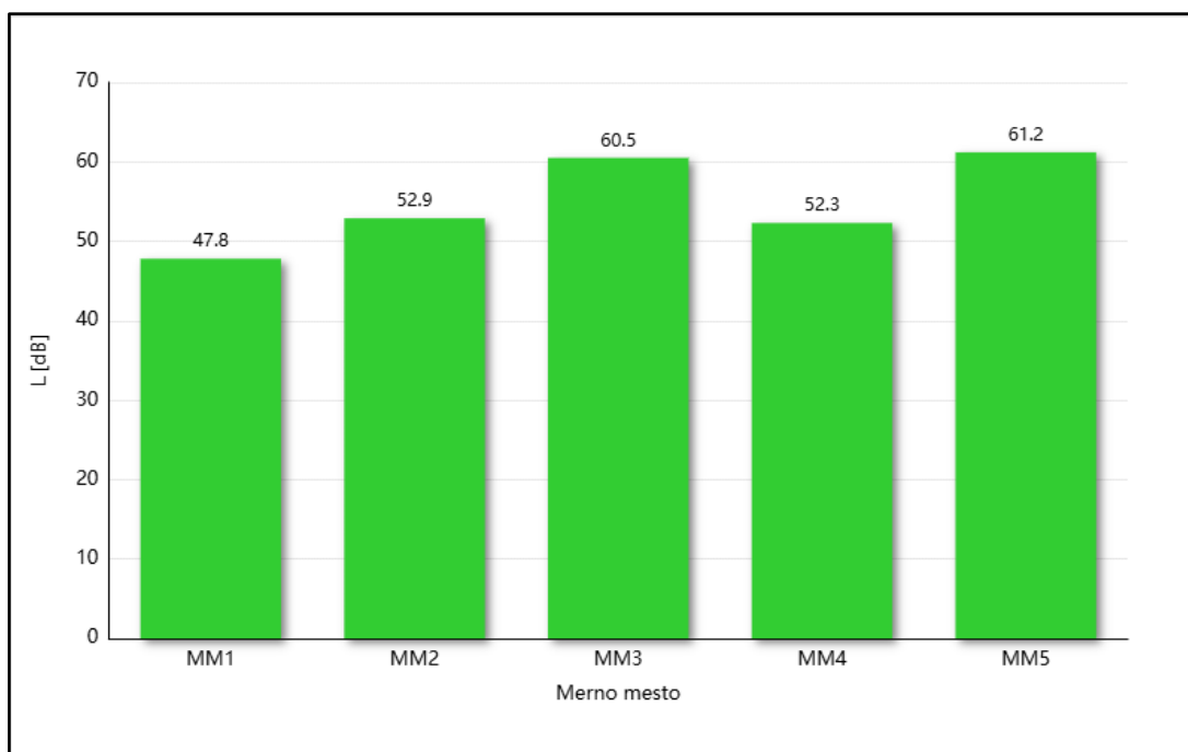
Grafik 5.7. - Dnevni period merenja 2 - Ekvivalentni nivoi buke - decembar 2025. godine
