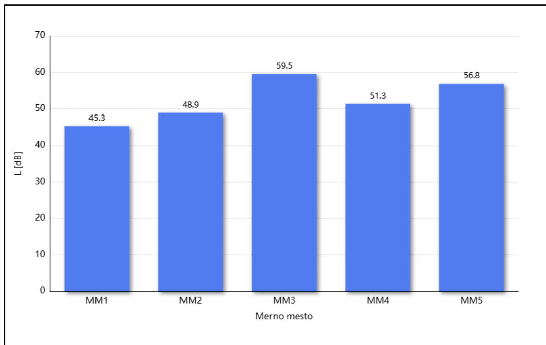
Grafik 5.8. - Večernji period merenja - Ekvivalentni nivoi buke - decembar 2025. godine
